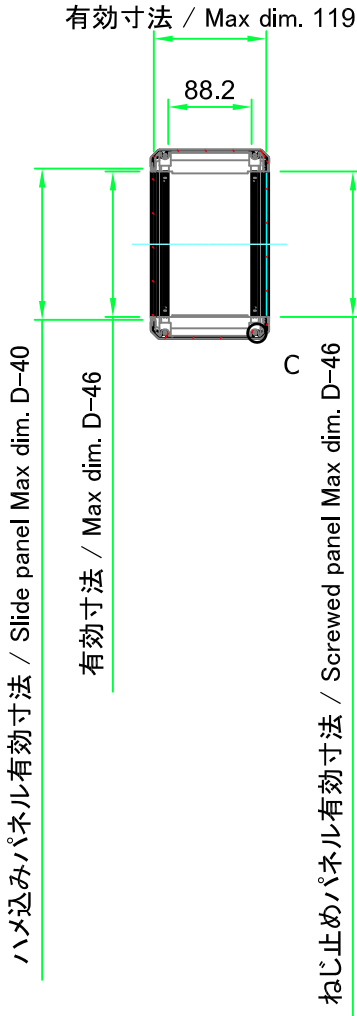
C : フレーム拡大図 Frame cross-section
